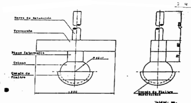
FIGURA 1 - MUESTRA DE ENSAYO "PASTOR"
