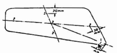
FIGURA 2 - LOCALIZACION DE LOS PUNTOS DE IMPACTO PARA V.S.T. PLANOS
