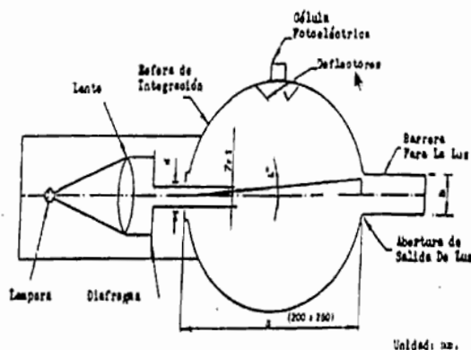
FIGURA 2 - CELULA FOTOELÉCTRICA
