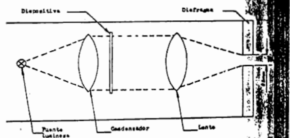
FIGURA 2 - DISPOSICIÓN ÓPTICA DEL PROYECTOR
