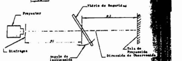
FIGURA 4 - DISPOSICIÓN DEL EQUIPO PARA EL ENSAYO DE DISTORSIÓN ÓPTICA
