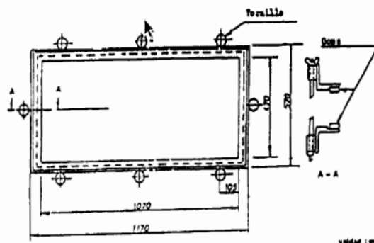
FIGURA 1 - MUNDO DE ENSAYO "PHANTOM"
