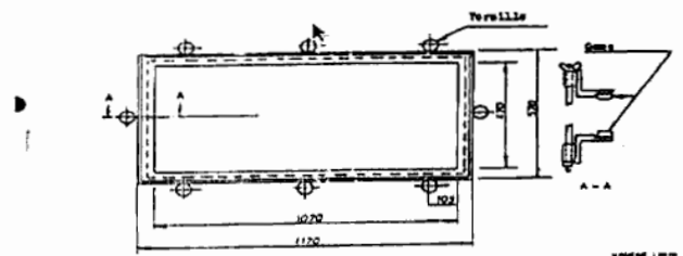
FIGURA 1 - MUESTRA DE ENSAYO "PASTOR"
