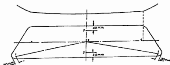
FIGURA 3 - LOCALIZACION DE LOS PUNTOS DE IMPACTO PARA V.S.T. CURVOS
