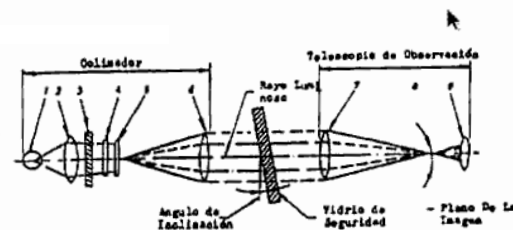
FIGURA 3.- EQUIPO PARA VERIFICACION CON COLIMADOR
