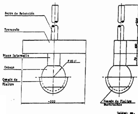
FIGURA 1 - MUNDO DE ENSAYO "PHANTOM"
