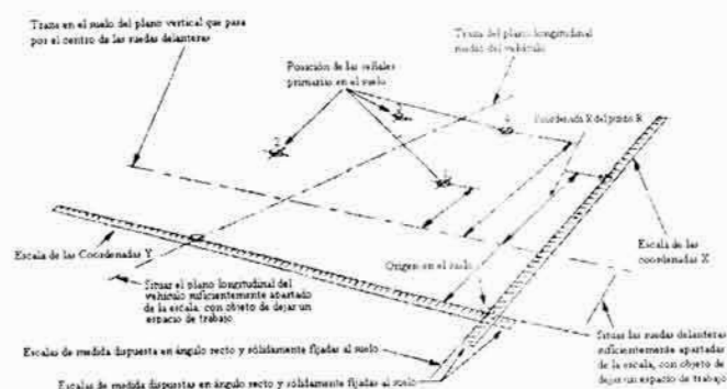
Figura 3 Área de medición horizontal
