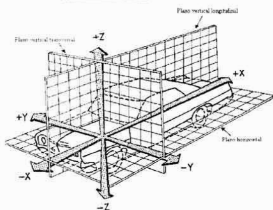
Figura 2 Sistema de referencia tridimensional
