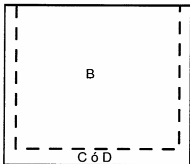
FIGURA 3. Zonas del vidrio para laterales delanteros
